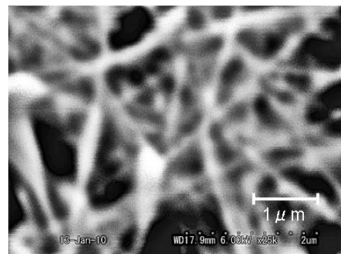
図3 試作したポリアミド酸繊維の電子顕微鏡写真
